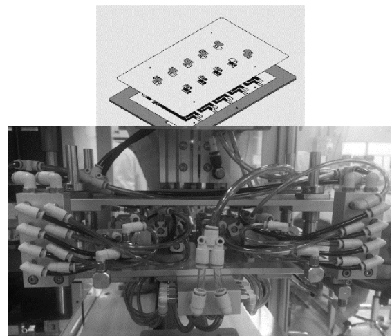
รูปที่ 3 บอร์ดสำหรับยึดตำแหน่ง Bare ให้คงที่
