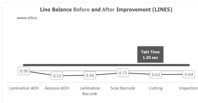
รูปที่ 9 สมดุลสายการผลิตก่อนและหลังปรับปรุงของสายที่ 5(C+D)
