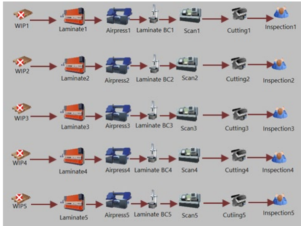
รูปที่ 10 แบบจำลองสถานการณ์หลังการปรับปรุง
