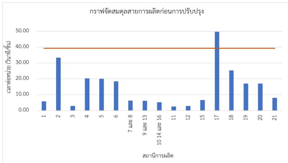
ภาพที่ 3 การจัดสมดุลสายการผลิตก่อนการปรับปรุง
