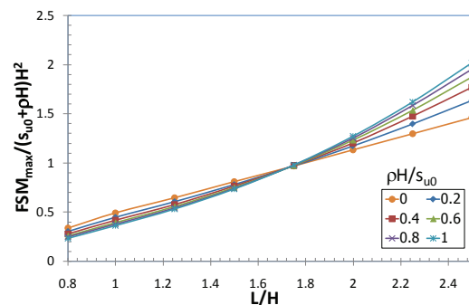
รูปที่ 14 ผลเฉลยโมเมนต์สูงสุดที่ pH/s_{u0} = 0 - 1
