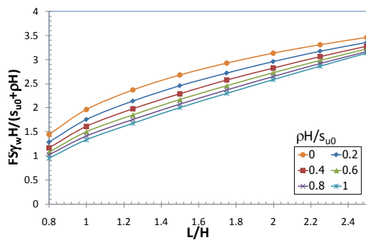
รูปที่ 10 ผลเฉลยตัวเลขเสถียรภาพที่ pH/s_{u0} = 0 - 1
