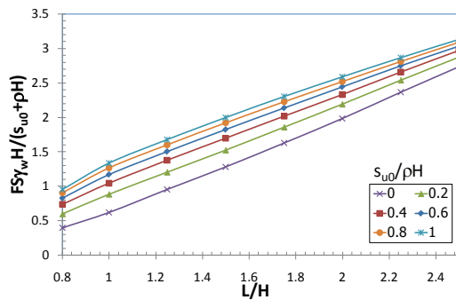
รูปที่ 11 ผลเฉลยตัวเลขเสถียรภาพที่ s_{u0}/pH = 0 - 1
